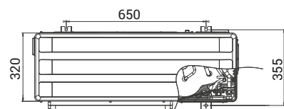
AONG36KBTV / AONG36KRТА
