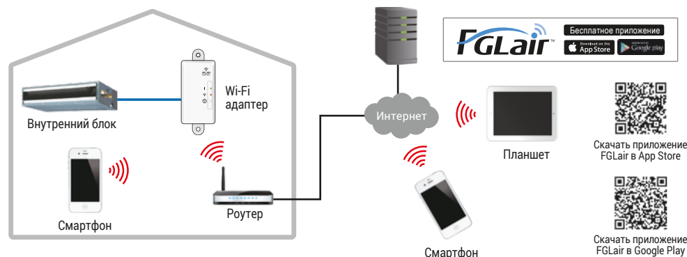
USB Wi-Fi адаптер для внутреннего блока сплит-системы UTY-TFSXF2
